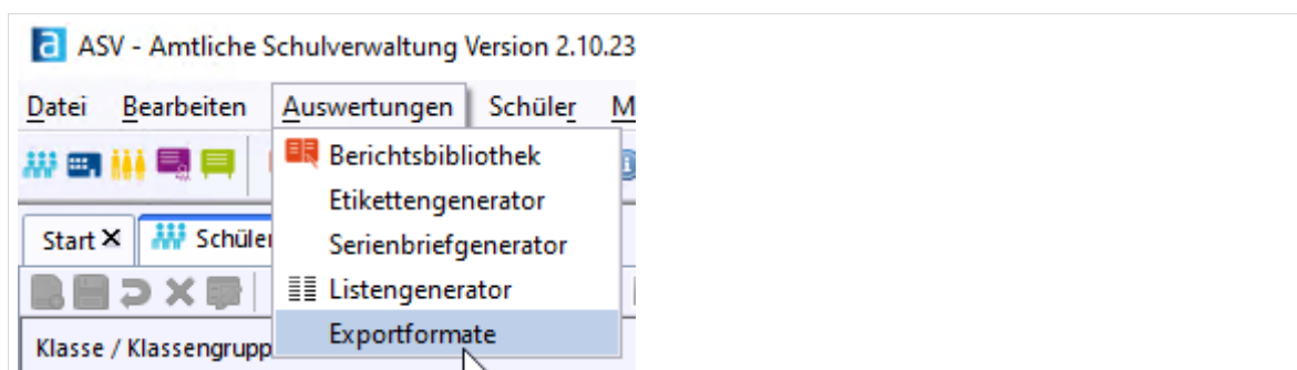
Abb. 10: ASV-BW Exportformate
