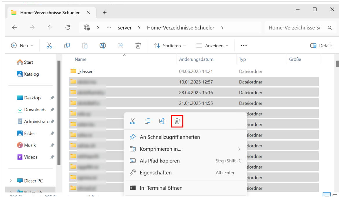
Abb. 9: Homelaufwerke leeren
