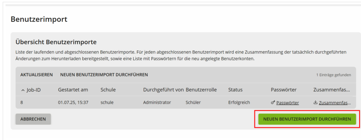
Abb. 35: Neuer Import
