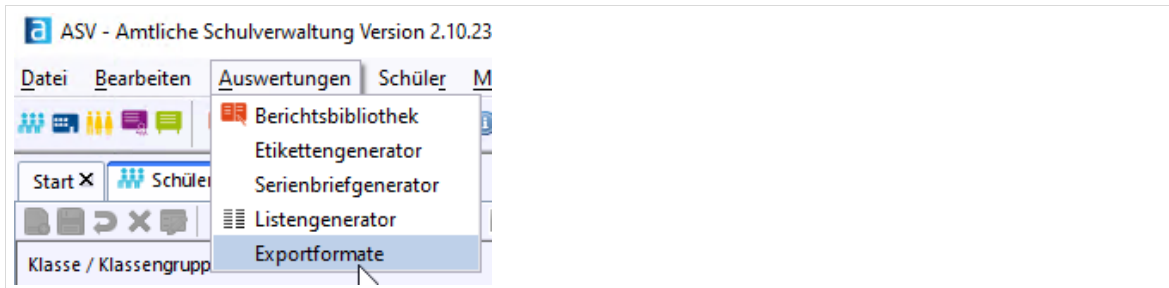
Abb. 31: ASV-BW Exportformate
