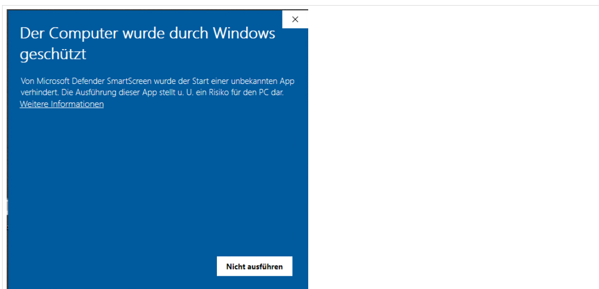
Abb. 1: Windows-Defender Warnung
