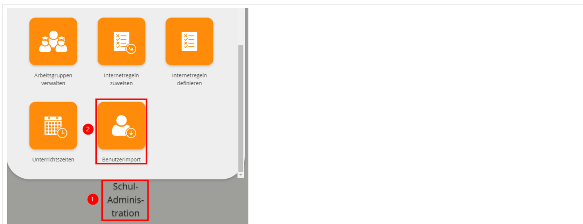
Abb. 17: Neuer Benutzerimport
