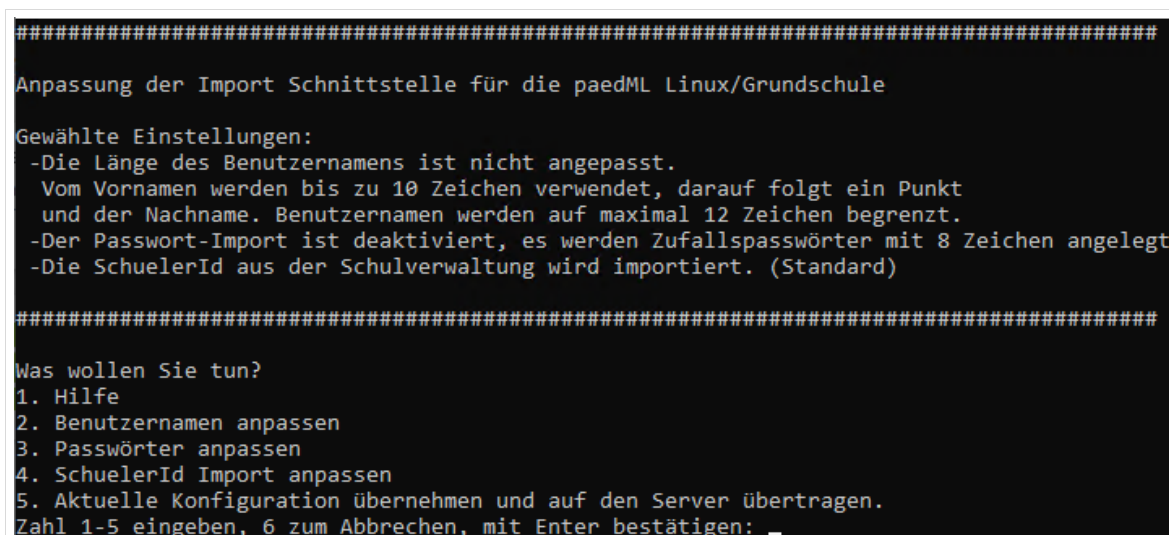
Abb. 30: benutzer-import-config.exe Menü
