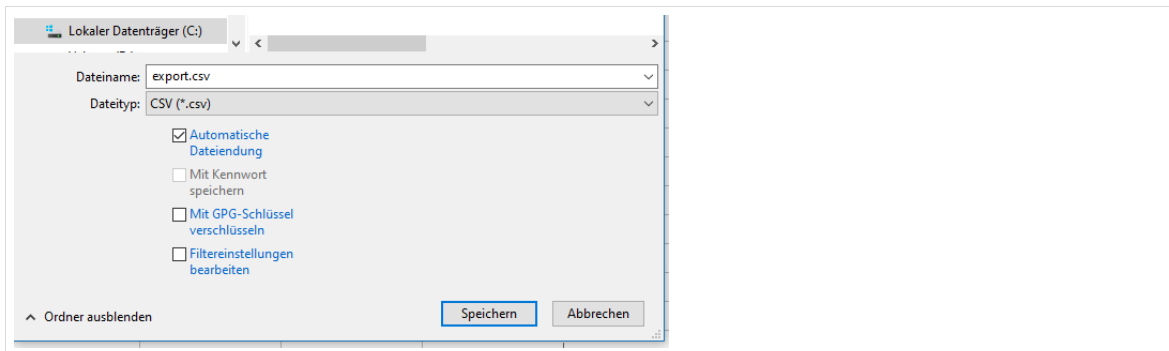
Abb. 28: CSV-Datei –abspeichern
